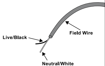
Hard wiring
